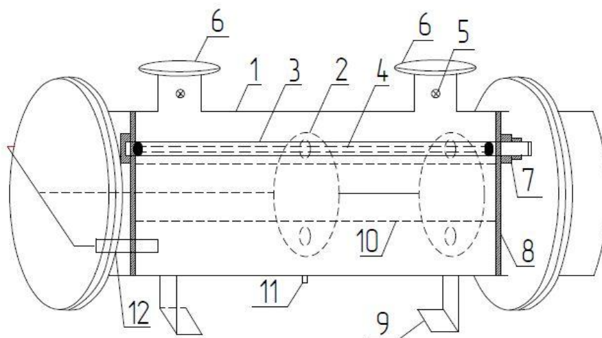
Рис. 1. Конструкция системы КИТ УФО
